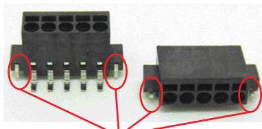
ホールダウン
